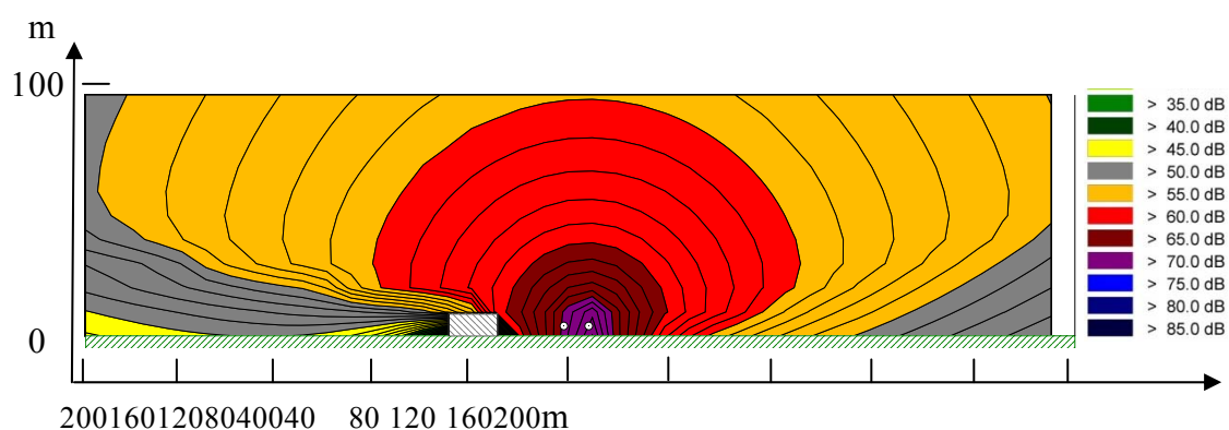
图 5.3-2 青茅至鹧鸪江增建二线路段夜间等声级曲线（4m 高路堤）
