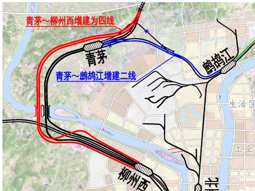
青茅至柳州西增建为四线工程示意图
