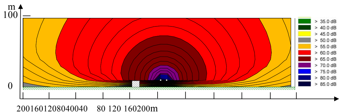
图 5.3-3 青茅至鹧鸪江增建二线路段昼间等声级曲线（10m 高桥梁）
