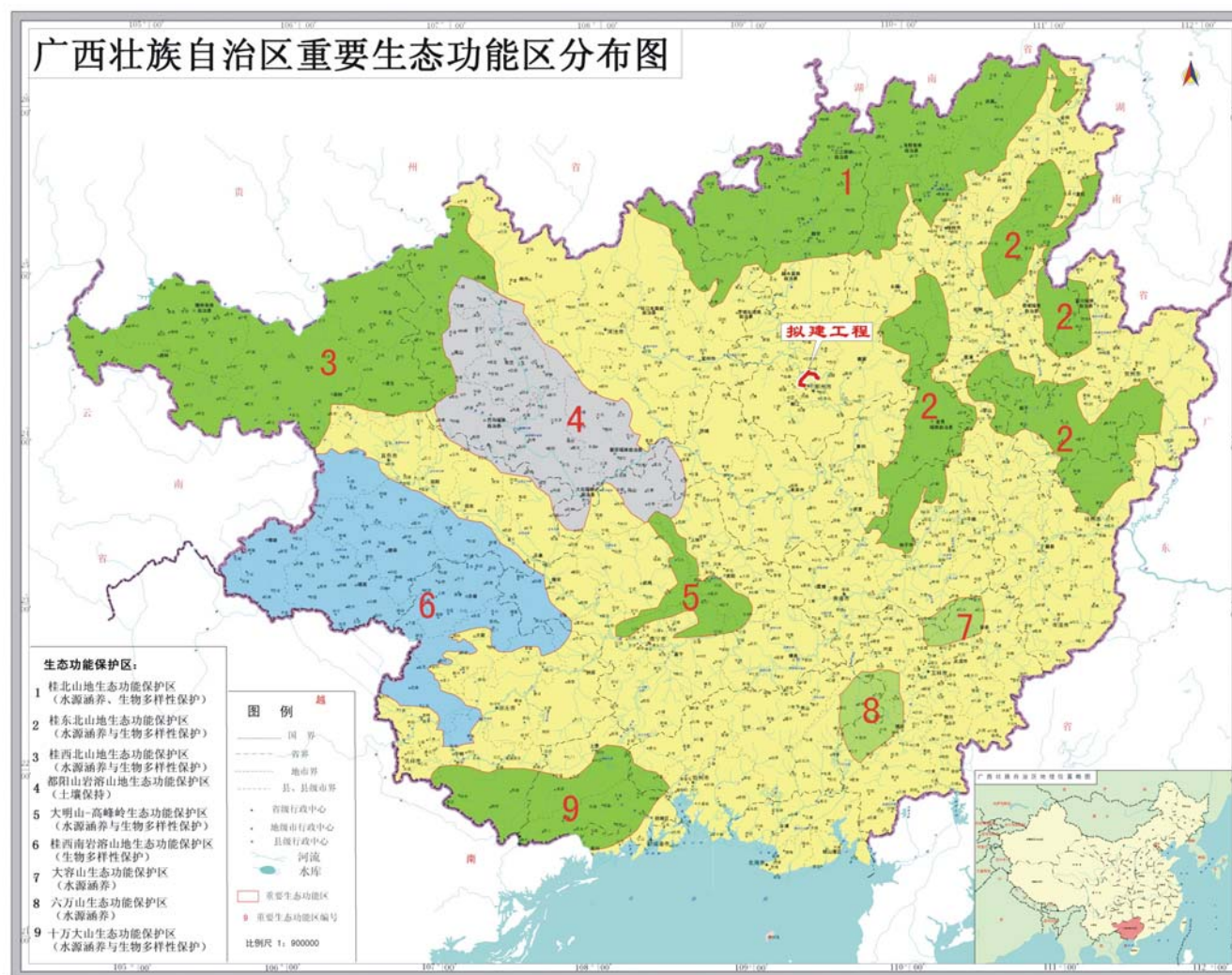
图 4.2-3 工程与广西自治区生态功能区域的位置关系图
