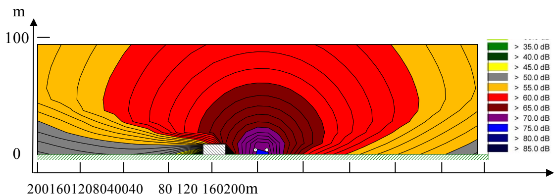
图 5.3-1 青茅至鹧鸪江增建二线路段昼间等声级曲线（4m 高路堤）
