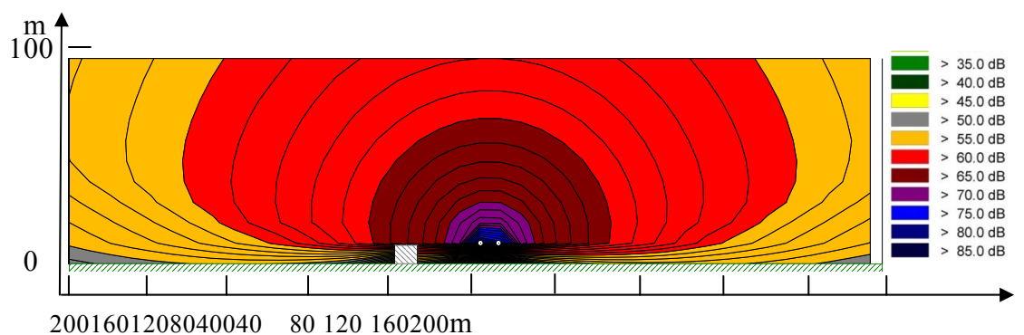
图 5.3-4 青茅至鹧鸪江增建二线路段夜间等声级曲线（10m 高桥梁）
