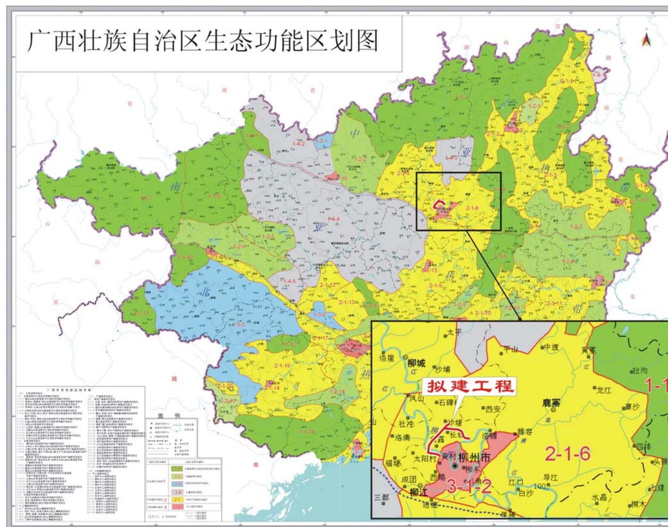
图 4.2-2 工程与广西自治区生态功能区域的位置关系图
